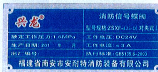
ZSXF-125-D(对夹式)
