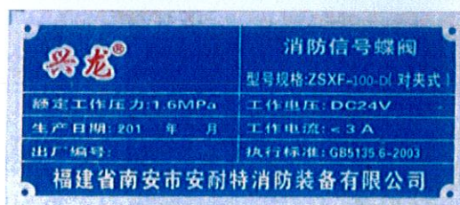
ZSXF-100-D(对夹式)
