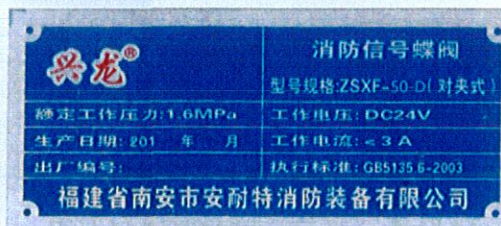
ZSXF-50-D(对夹式)
